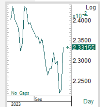
PTTGC/SET
