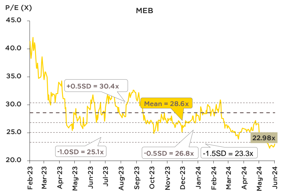
Fig 2. PE BAND
