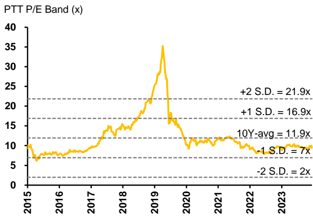
Fig. 5: PER Band
